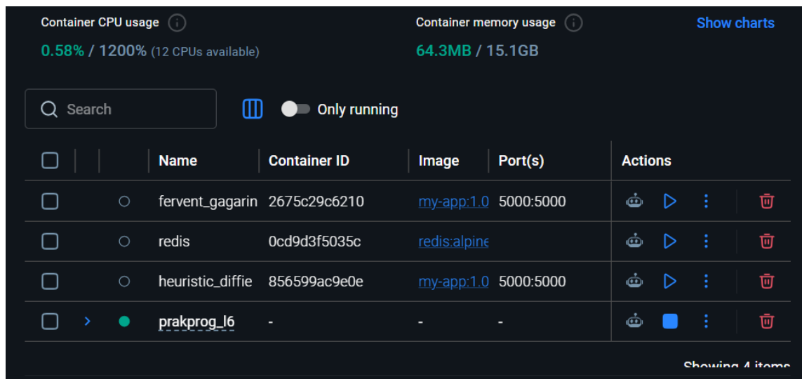
Rysunek 6: Uruchomiony kontener - Docker Desktop
